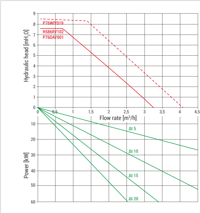
Diagramma di portata/potenza/prevalenza
