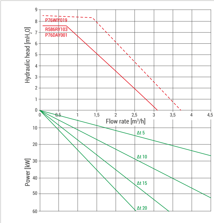
Diagramma di portata/potenza/prevalenza
