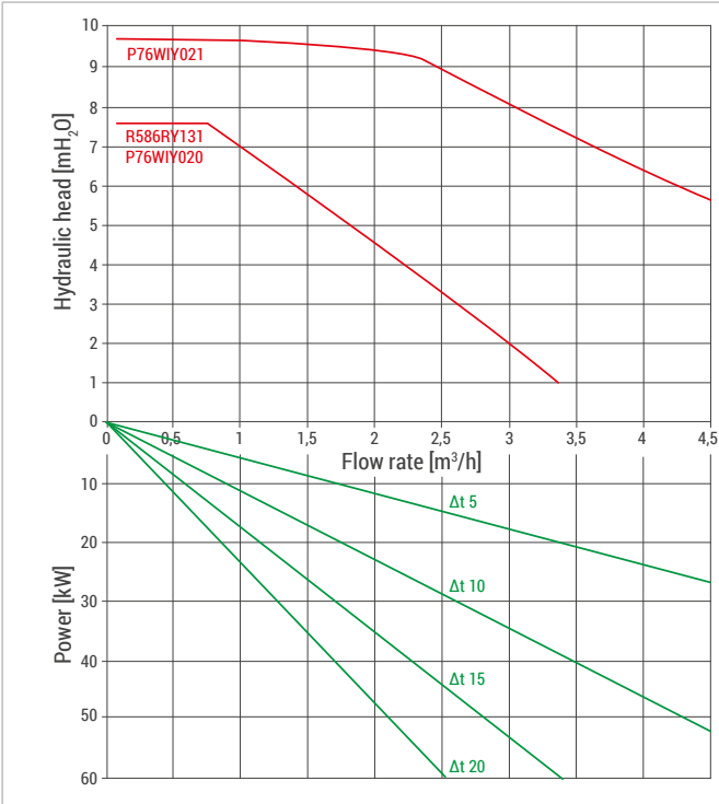
Diagramma di portata/potenza/prevalenza
