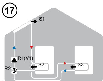
Solare + 2. accumuli con valvola
