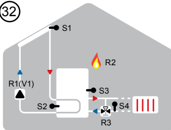
Solare con termostato e pre-riscaldamento
