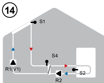
Solare + scamb.
