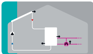
Solare con scambiatore con funzione aggiuntiva aumento ritorno
