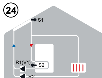
Solare + raffreddamento 2
