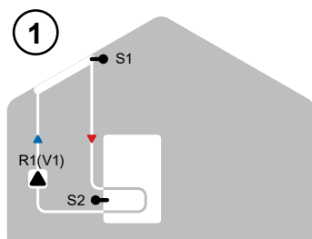
Solare
