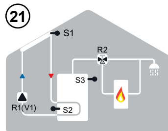
Solare + termostato come valvola
