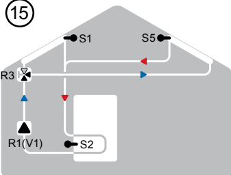
Solare + 2 collettori
