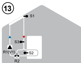
Solare + bypass
