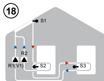
Solare + 2. accumuli + pompa
