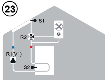
Solare + raffreddamento 1
