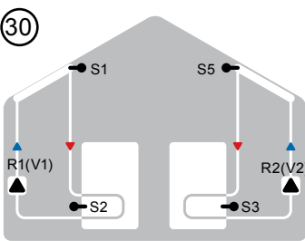
Doppio solare
