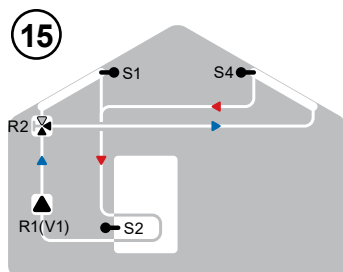
Solare + 2 collettori
