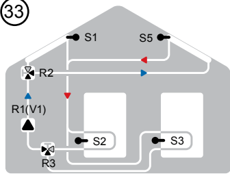
Solare est-ovest, 2 accumuli, 2 valvole
