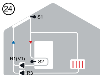
Solare + raffreddamento 2
