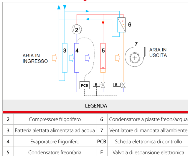
Figura 2 - Funzionamento termo igrometrico
