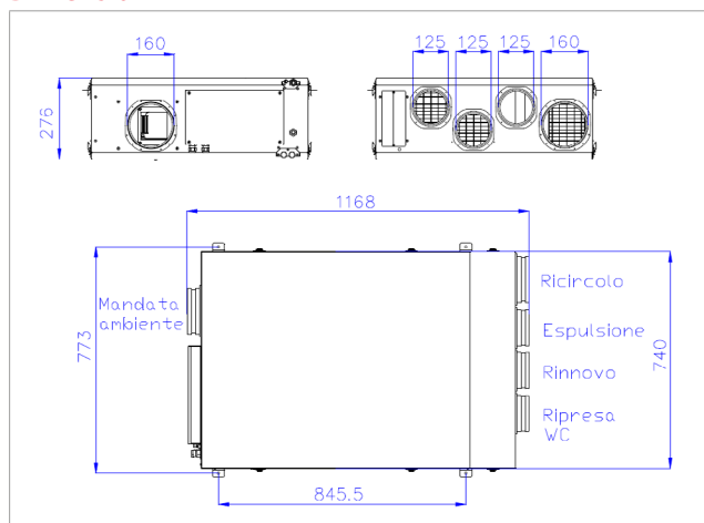
Figura 4 - Dimensioni in mm
