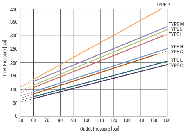
A221/A222 - STATIC OUTLET
