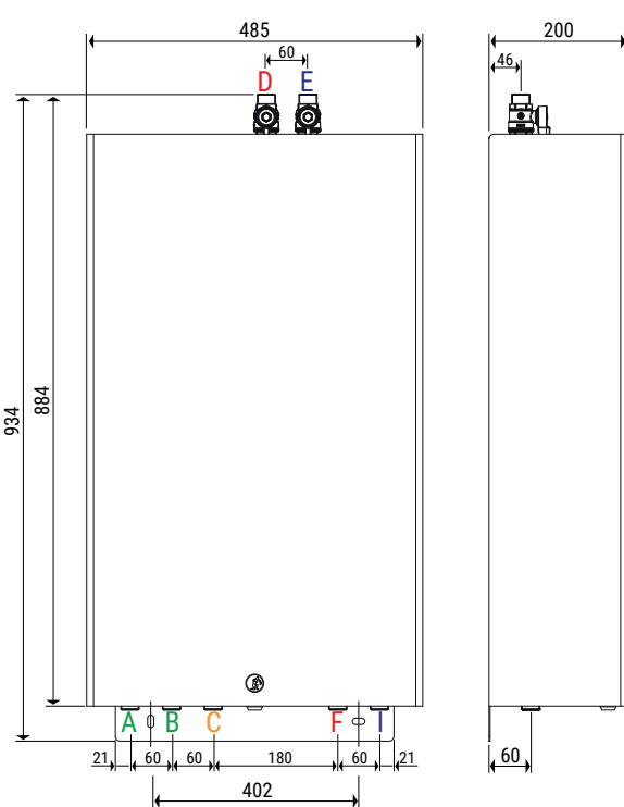
GE556-SM RADIATEUR, avec raccords par le haut, gabarit GE551Y097, isolation et coffret GE551Y194
