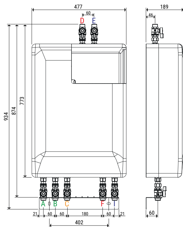
GE556-SM RADIATEUR, avec raccords par le haut, gabarit GE551Y097 et isolation
