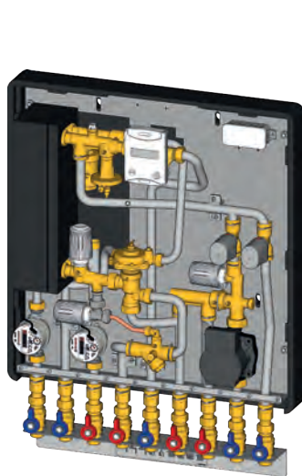
Raccordements primaires par le bas
