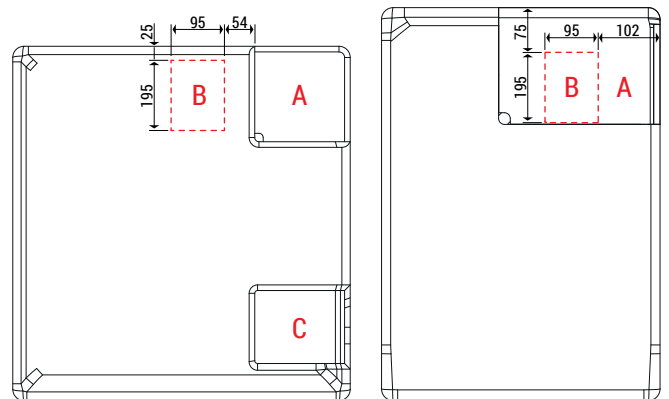
Isolation MTA version RADIATEUR Dimensions : 673x477x189 mm
