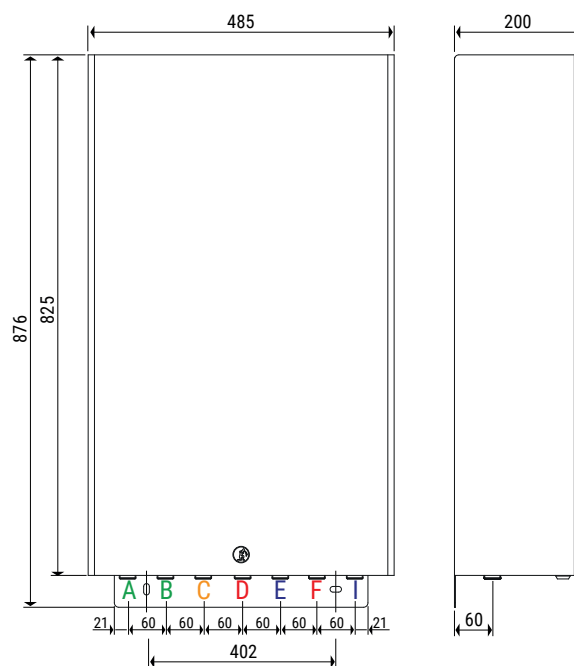
GE556-SM RADIATEUR, avec raccords par le bas, gabarit GE551Y097, isolation et coffret GE551Y194
