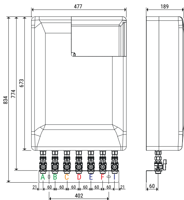
GE556-SM RADIATEUR, avec raccords par le bas, gabarit GE551Y097 et isolation
