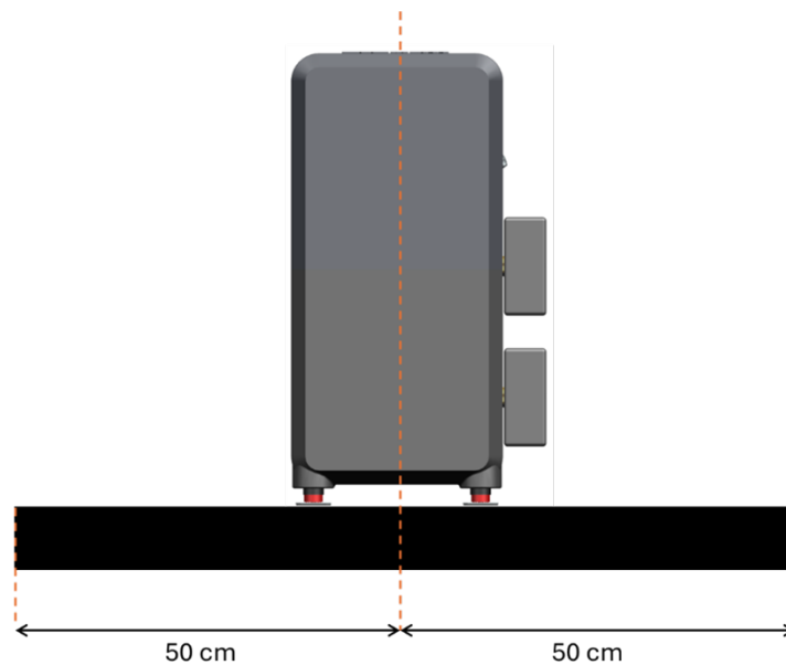
De HPM-WS op de montagerail
