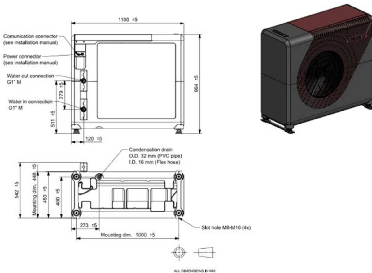
Afmetingen van de HPM-WS
