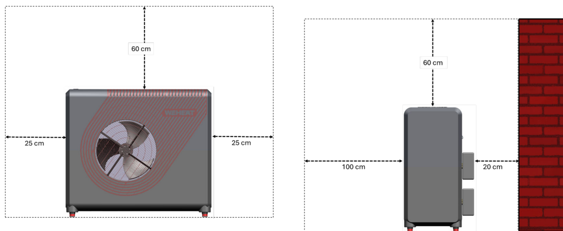
Afmetingen van de HPM-WS
