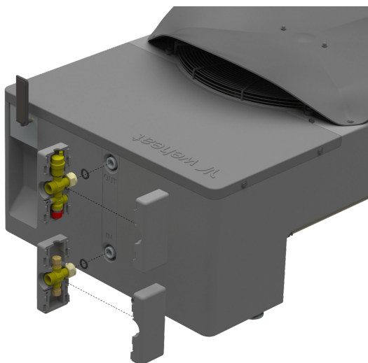
Montage van de appendage isolatie
