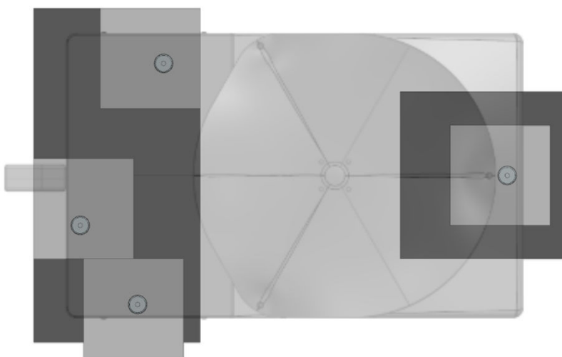
Tegellocatie (bovenaanzicht) - 4x tegels van 30x30cm (grijs) of 3x tegels van 50x50cm (zwart)
