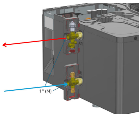
Aansluiting van de aan- en afvoer in de HPM-WB
